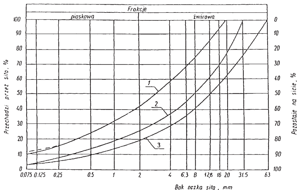
Rysunek 1. Pole dobrego uziarnienia kruszywa przeznaczonych na podbudowę wykonywane metodą stabilizacji mechanicznej 1-2 kruszywo na podbudowę zasadniczą (górną warstwę) lub podbudowę
